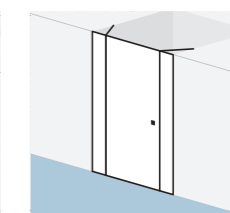
Pendeltür mit 2 Fest- feldern, Anschlag links oder rechts
